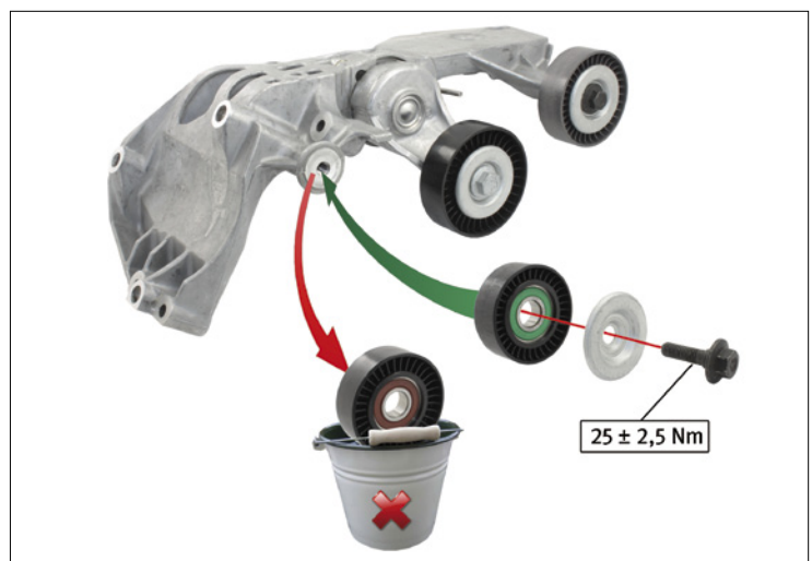
Figura 1: Unidad tensora 534 0243 10
