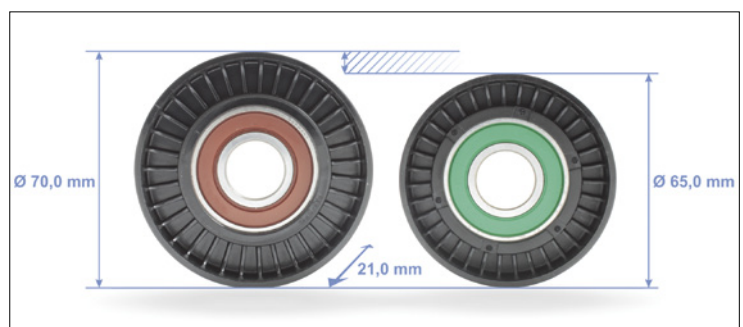
Figura 2: Polea de inversión 532 0404 30 para vehículos con motores gasolina (izquierda) y polea de inversión 532 0406 30 para vehículos con motores diésel (derecha)
