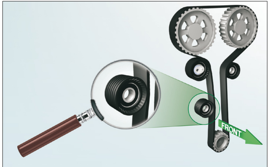
Fig 1: Recorrido de la correa y posiciones de las poleas en el motor F4R
